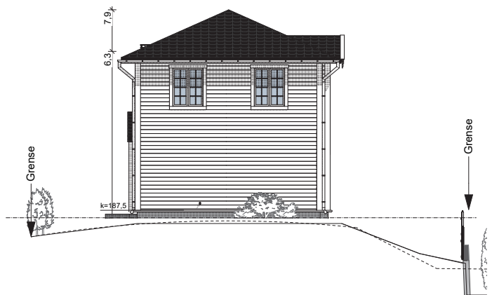
Fasade Nord
