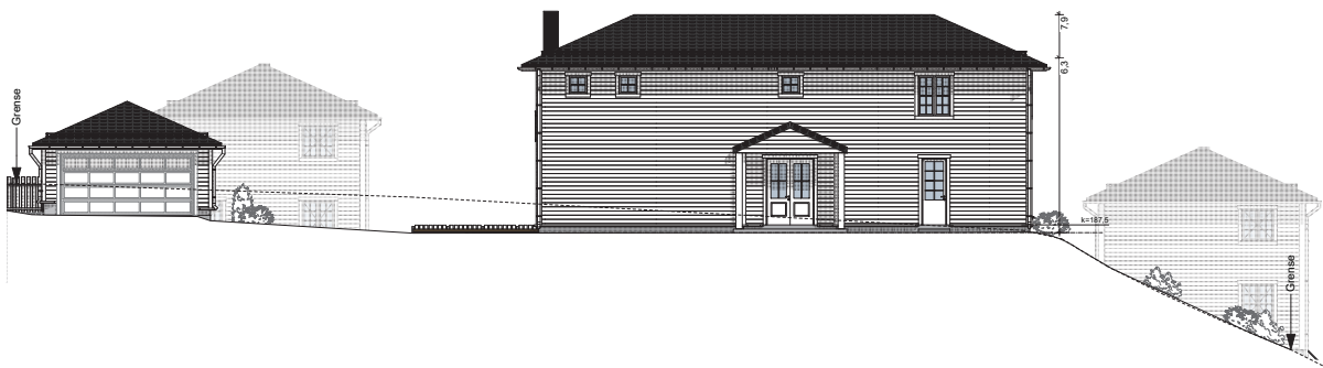
Fasade Øst
