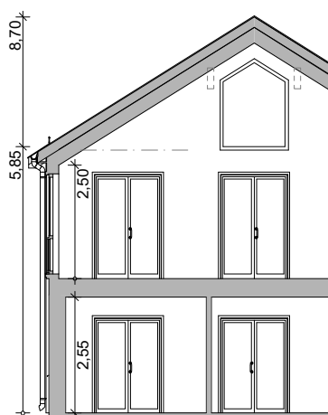
Snitt A 1:150
