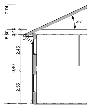
Snitt A
