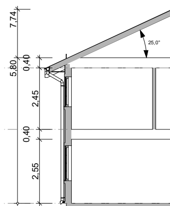
Snitt A 1:150
